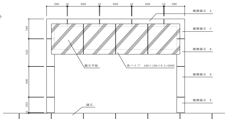
断面図
