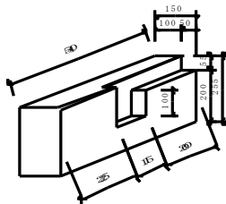
縁石B
