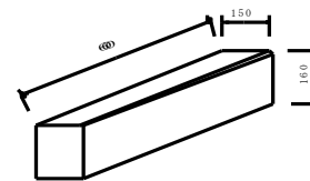
縁石D
