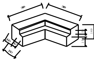
縁石C
